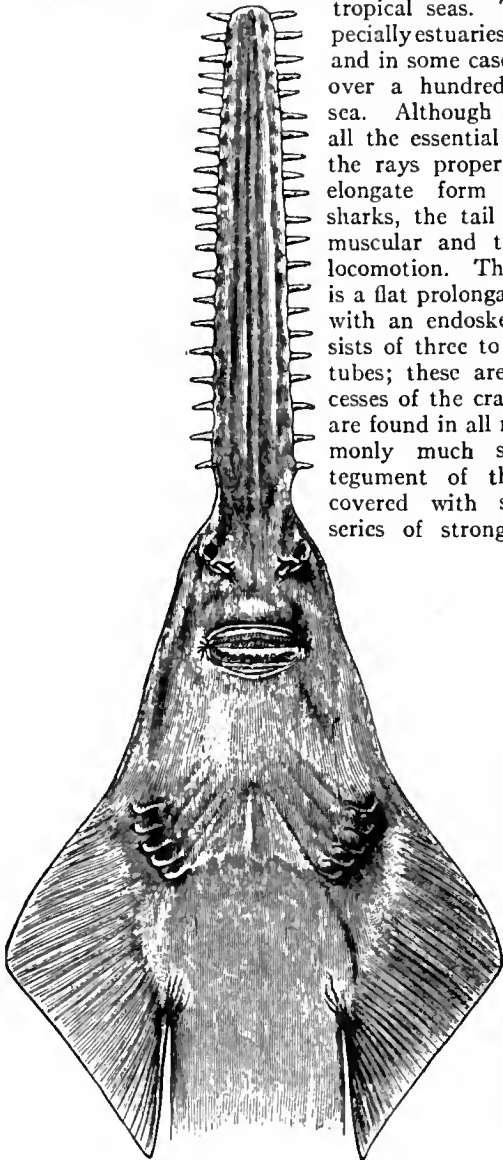
FIG. 1.— Pristis perrotletii .
