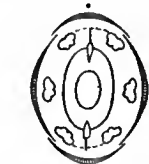
FIG. 5.— Oxyria .
