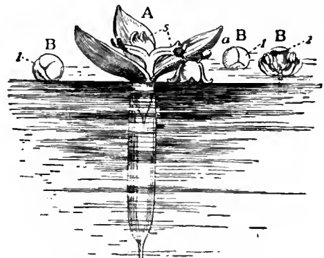
FIG. 4.— Vallisneria spiralis .
