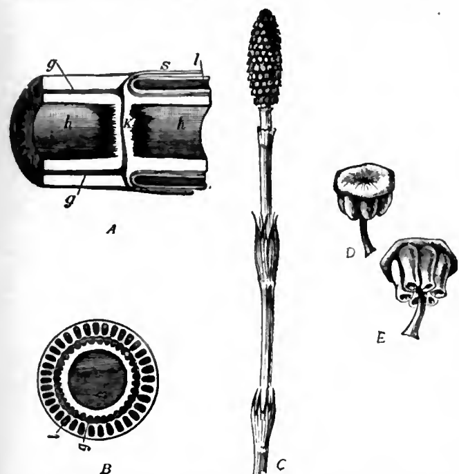
FIG. 3.— Equisetum maximum .
